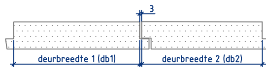
Doorsnede AA
