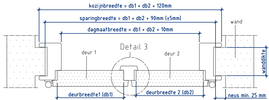
Doorsnede AA
