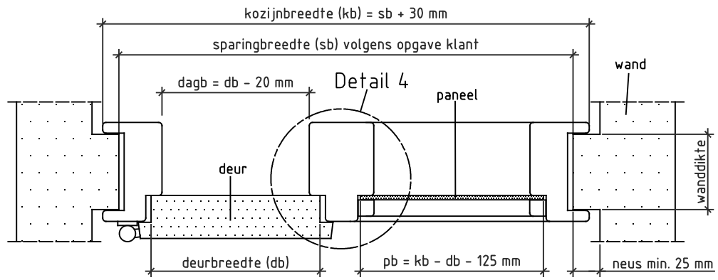
Doorsnede AA
