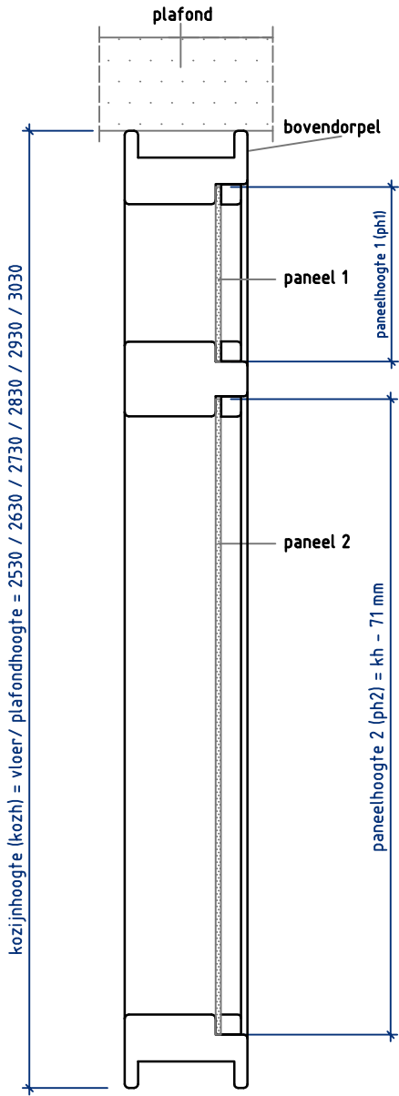
Doorsnede BB
