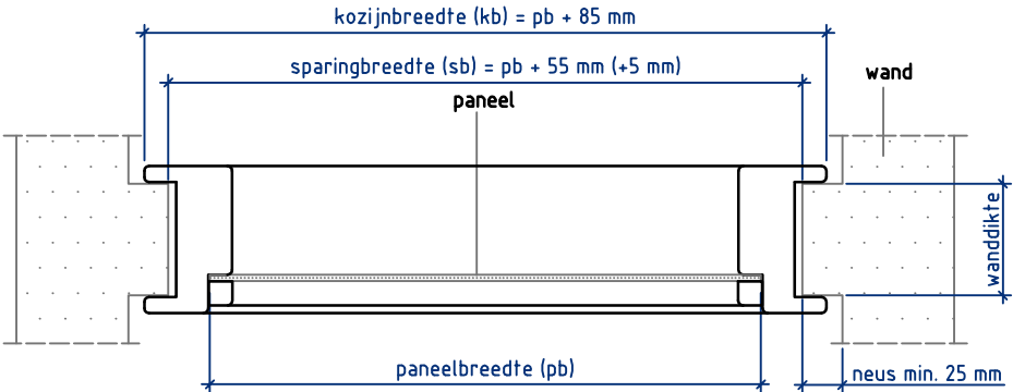
Doorsnede AA
