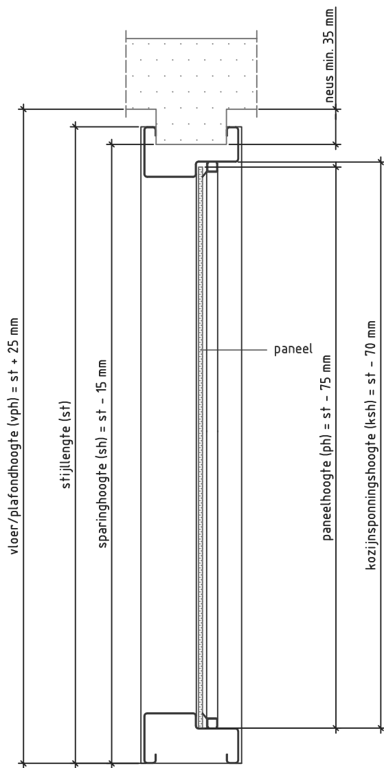
Doorsnede CC
