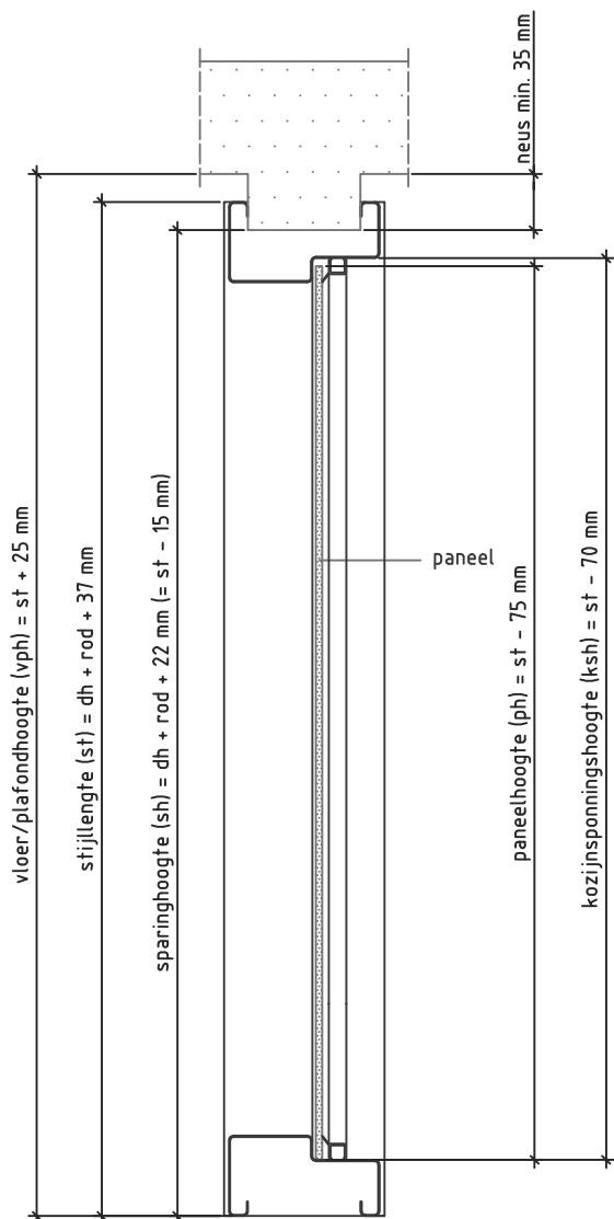
Doorsnede BB
