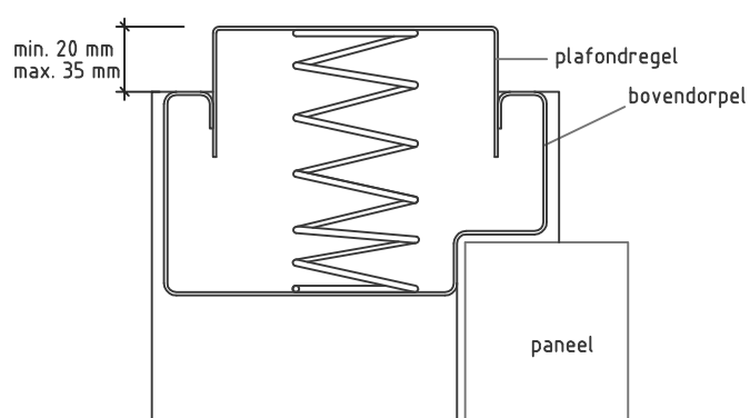
Optioneel plafondregel
