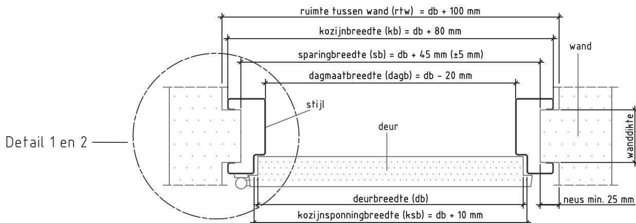
Doorsnede AA
