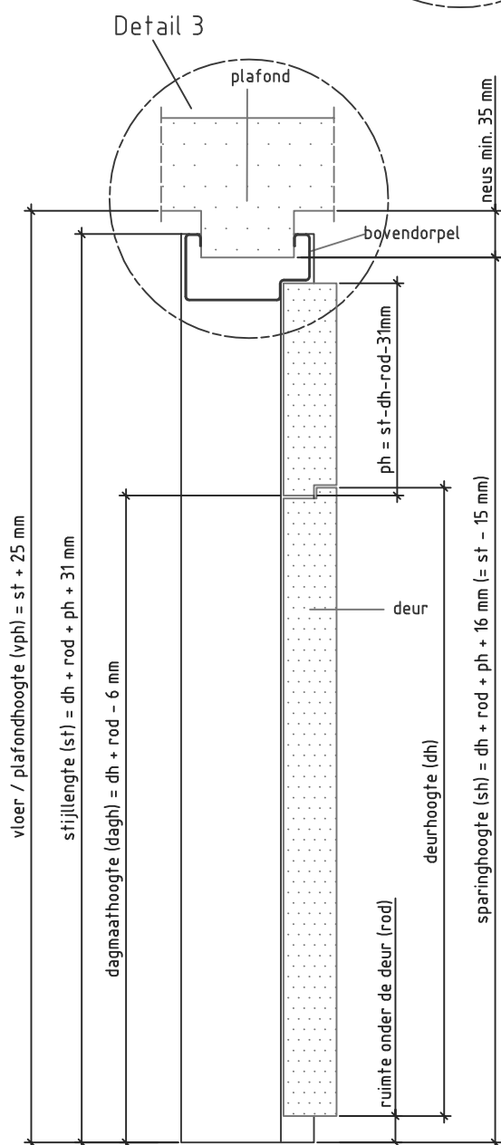
Doorsnede BB
