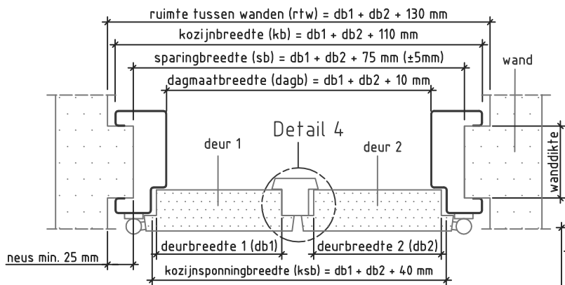
Doorsnede AA T-lat
