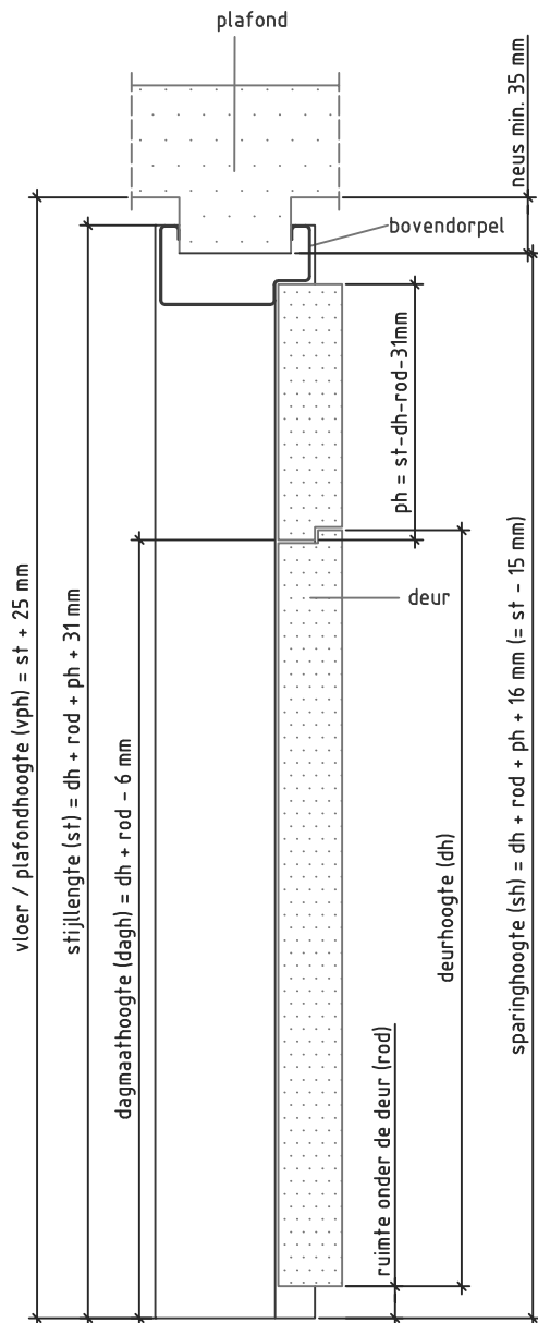
Doorsnede BB
