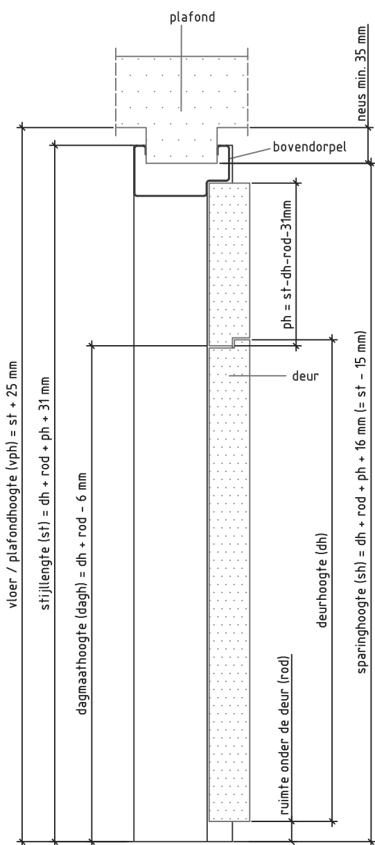
Doorsnede BB
