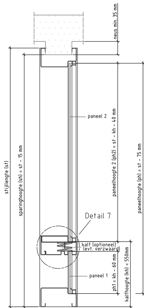
Doorsnede CC
