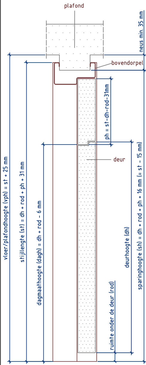
Doorsnede BB
