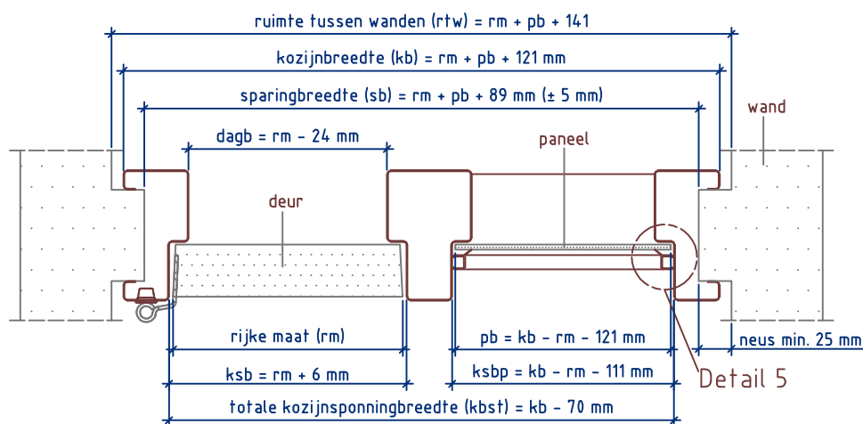
Doorsnede AA
