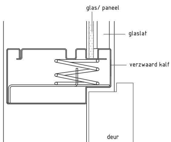
Detail 6: verzwaard kalf
