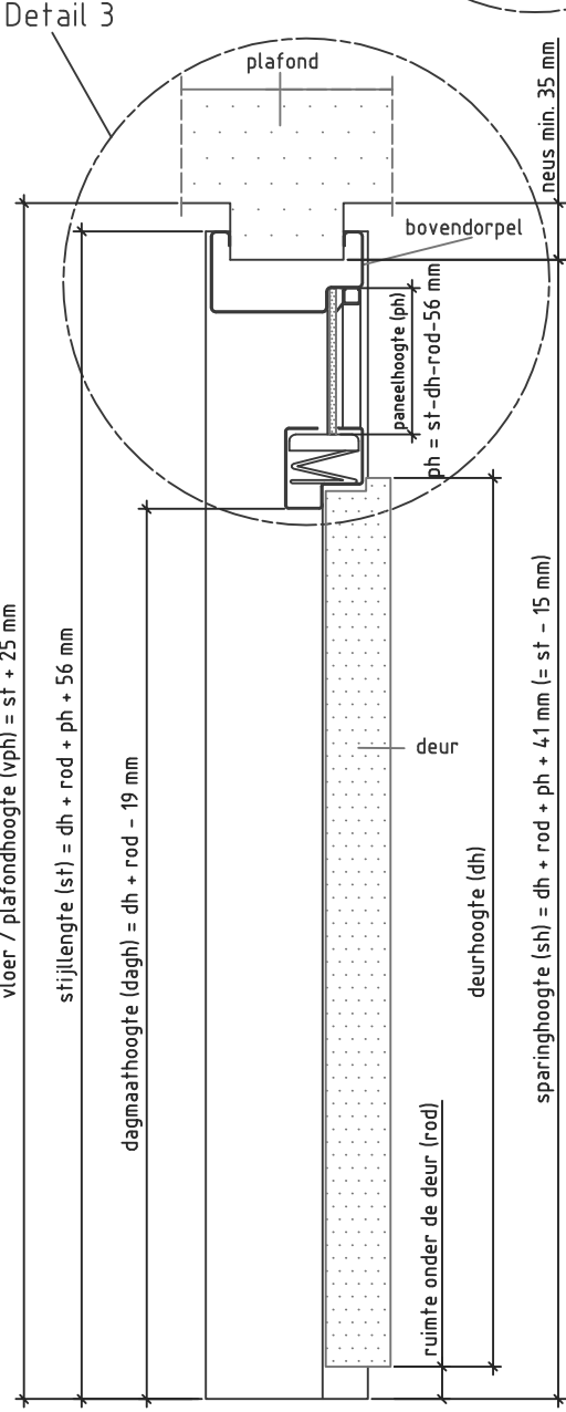
Doorsnede BB
