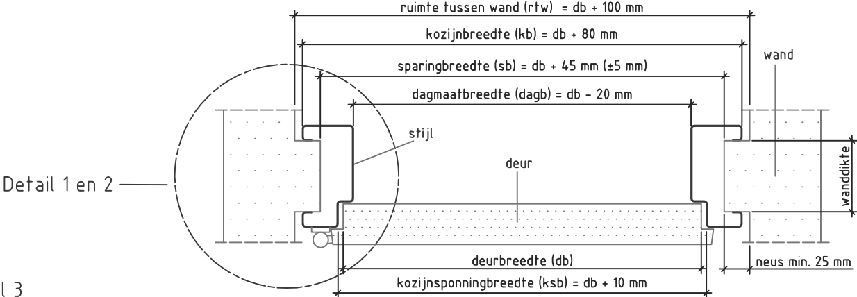
Doorsnede AA
