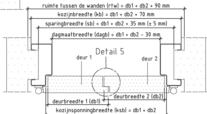
Doorsnede AA sponning/contrasponning
