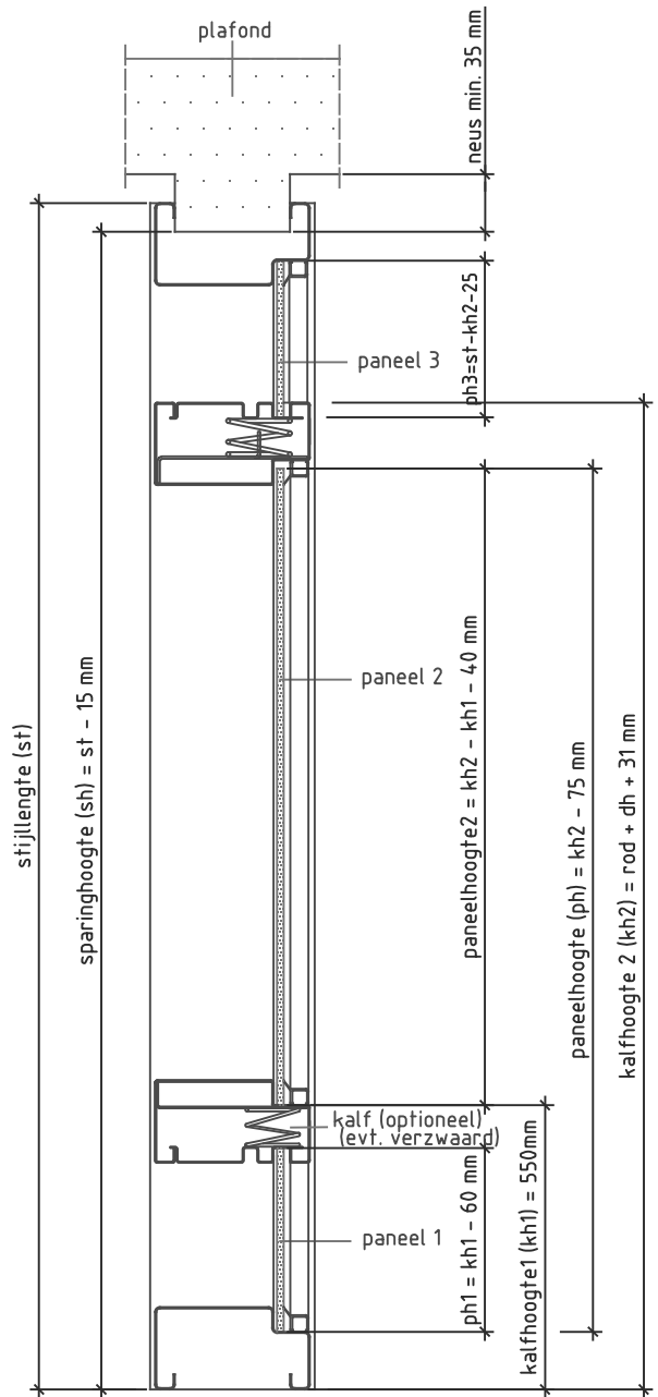
Doorsnede CC
