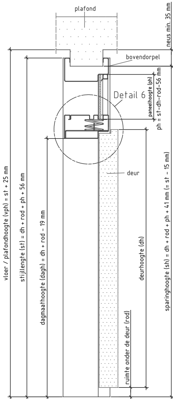
Doorsnede BB
