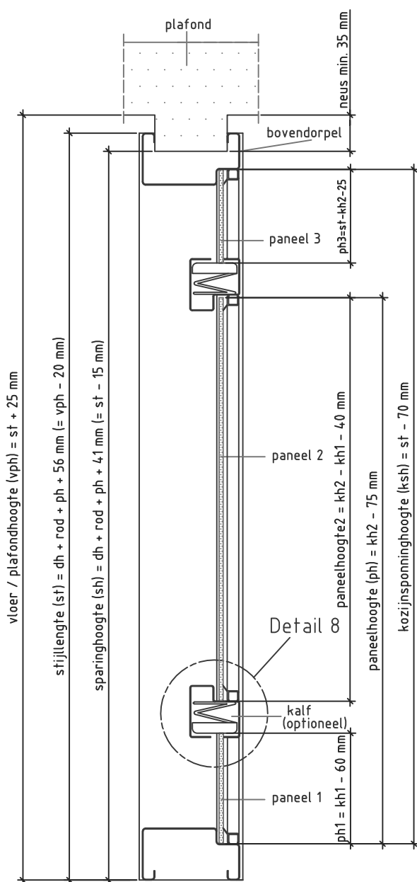
Doorsnede BB
