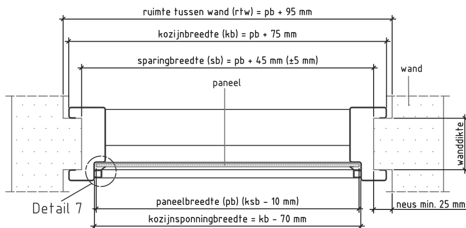
Doorsnede AA
