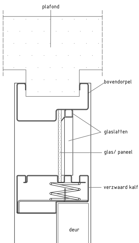
Detail 3: bovendorpel
