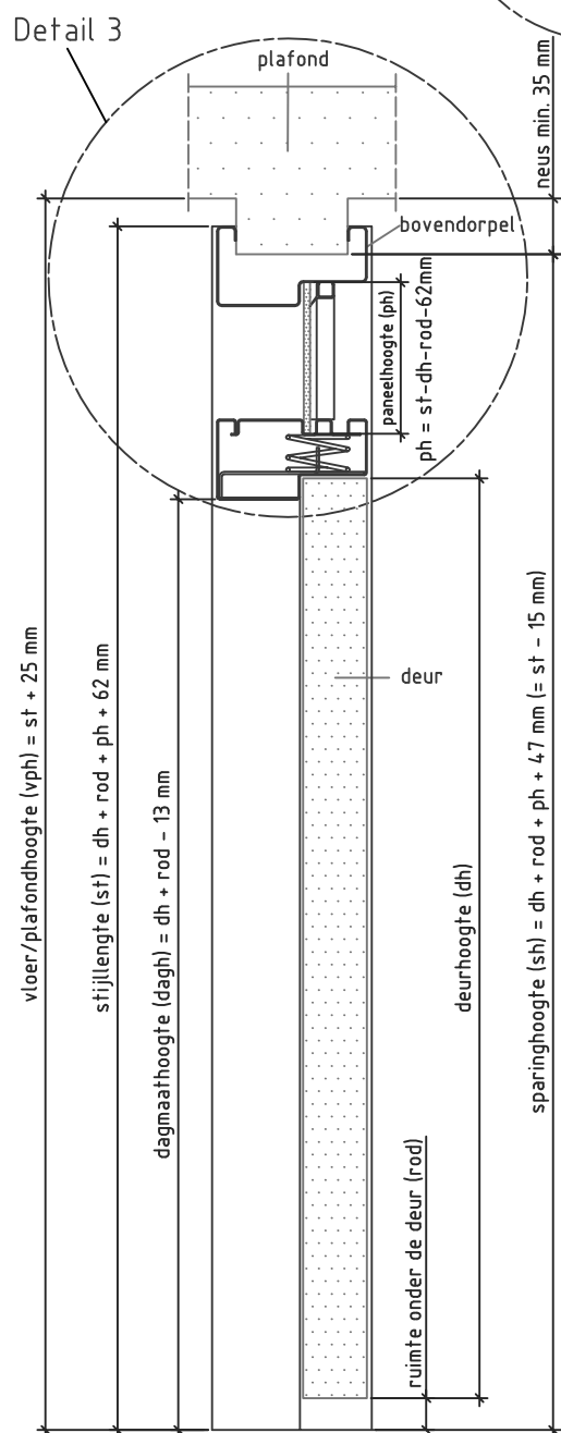
Doorsnede BB
