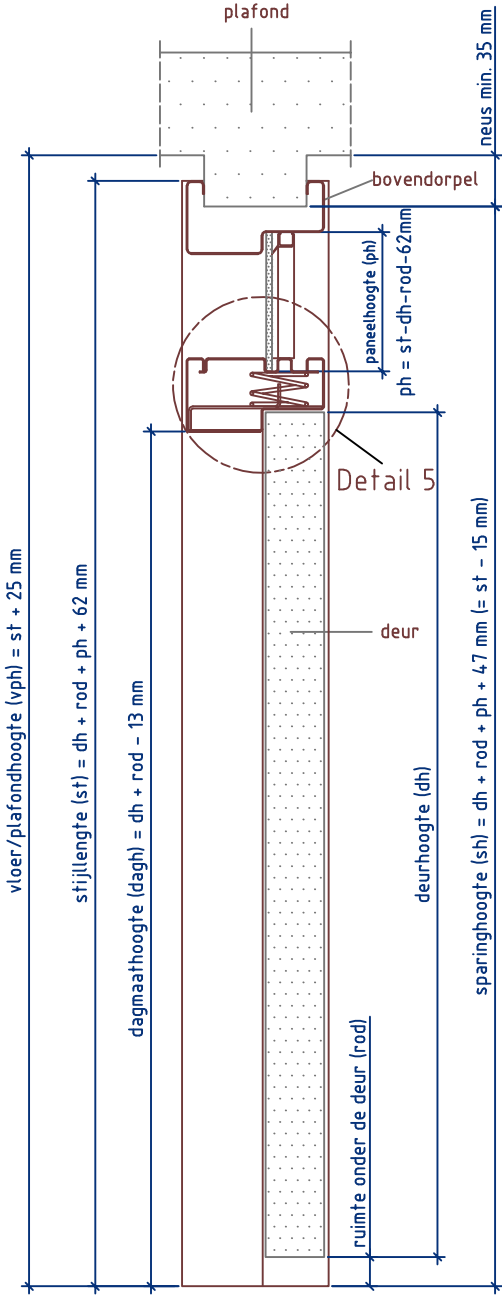
Doorsnede BB
