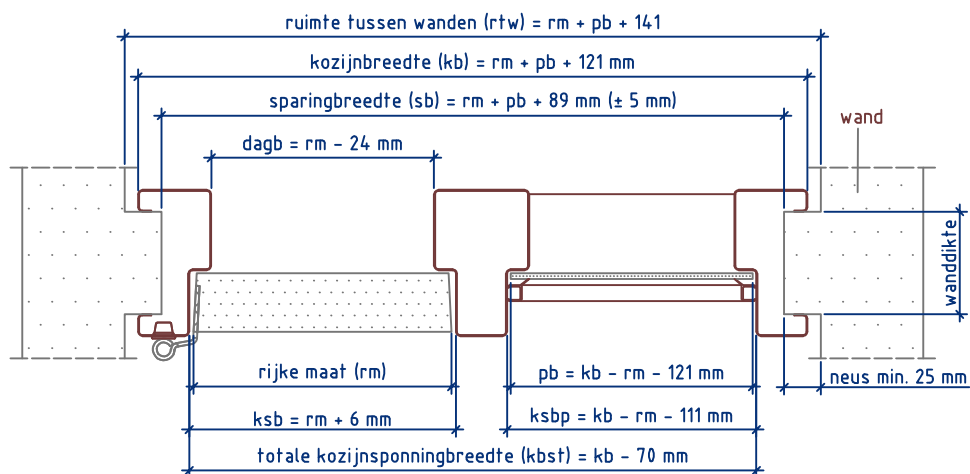
Doorsnede AA
