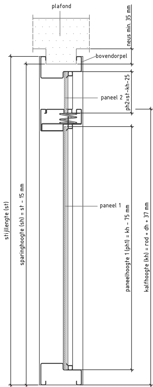
Doorsnede CC
