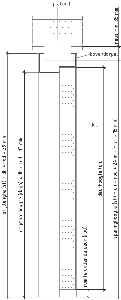
Doorsnede BB
