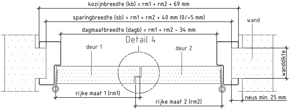
Doorsnede AA
