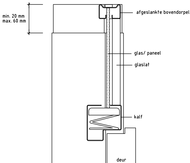
Detail 3: bovendorpel
