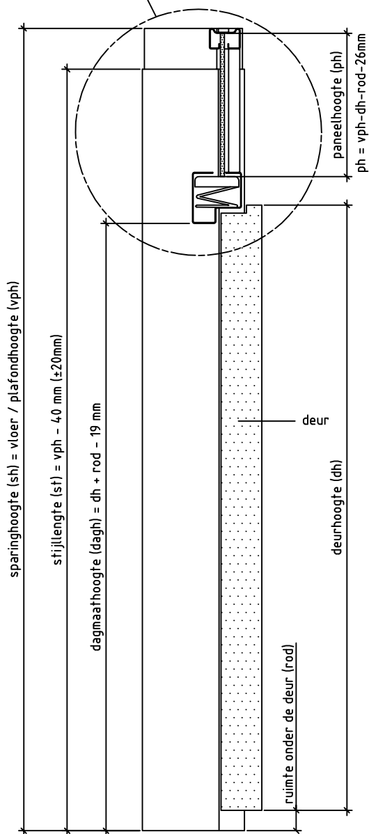
Doorsnede BB
