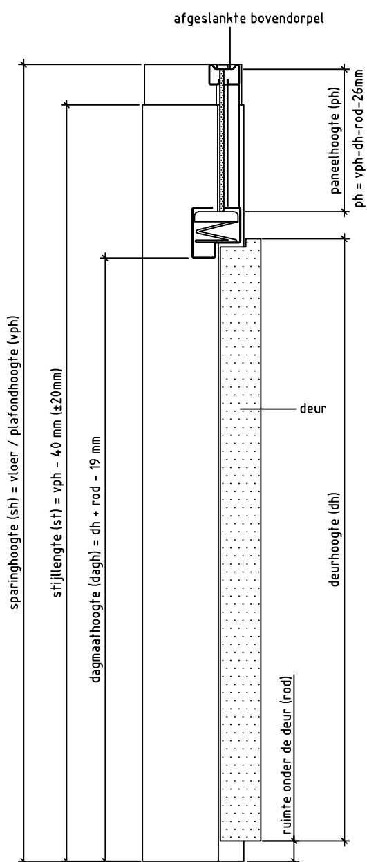
Doorsnede BB
