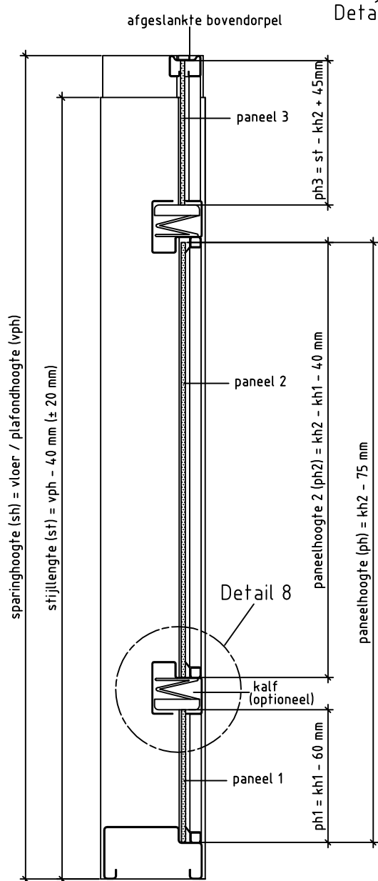
Doorsnede BB
