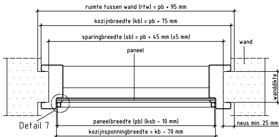
Doorsnede AA
