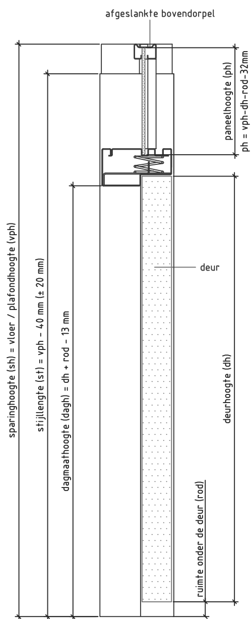
Doorsnede BB
