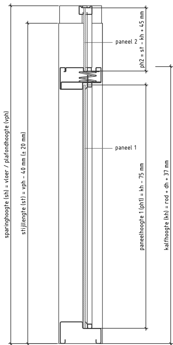
Doorsnede CC
