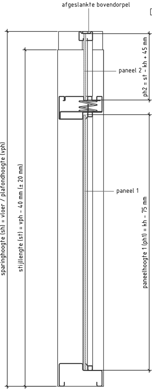
Doorsnede BB
