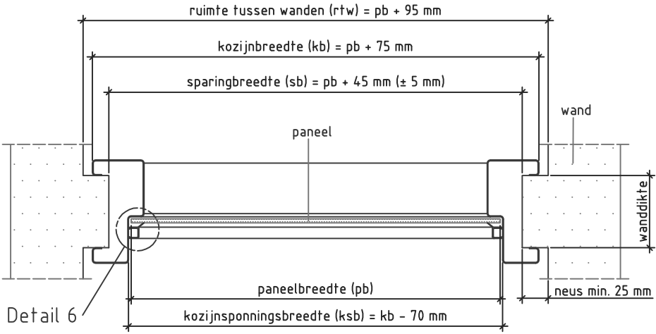
Doorsnede AA
