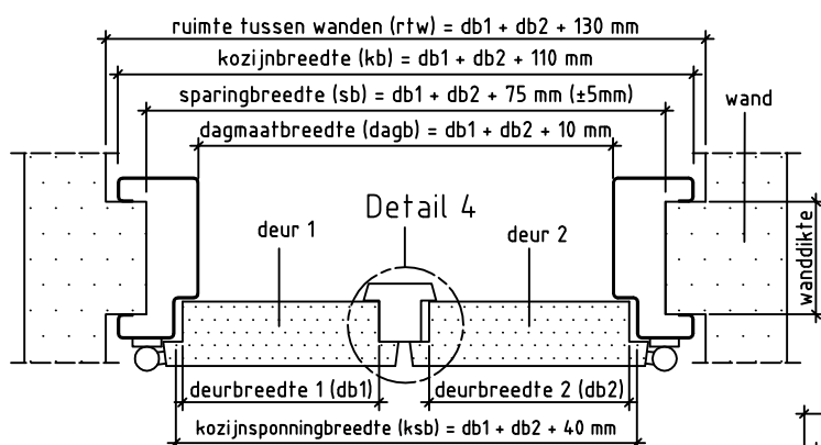
Doorsnede AA T-lat
