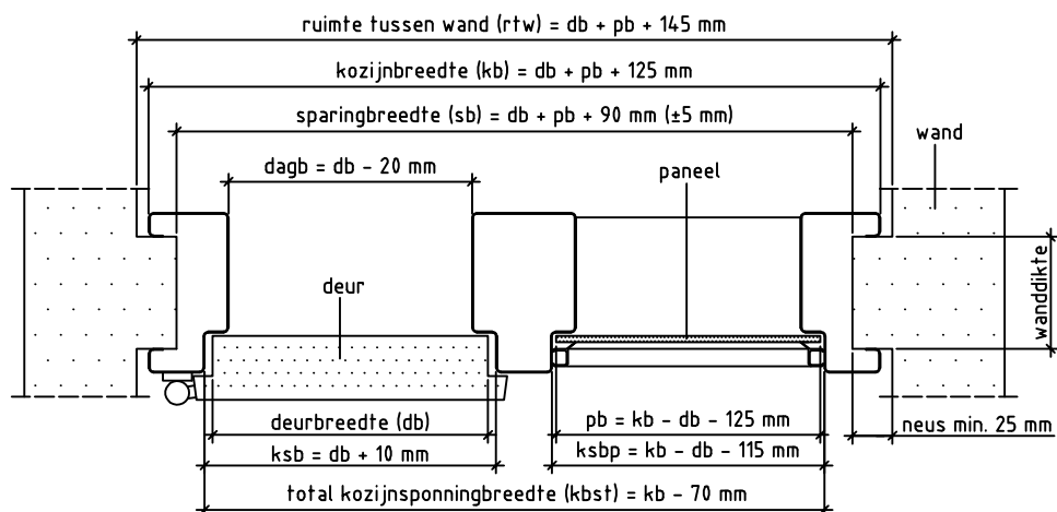
Doorsnede AA
