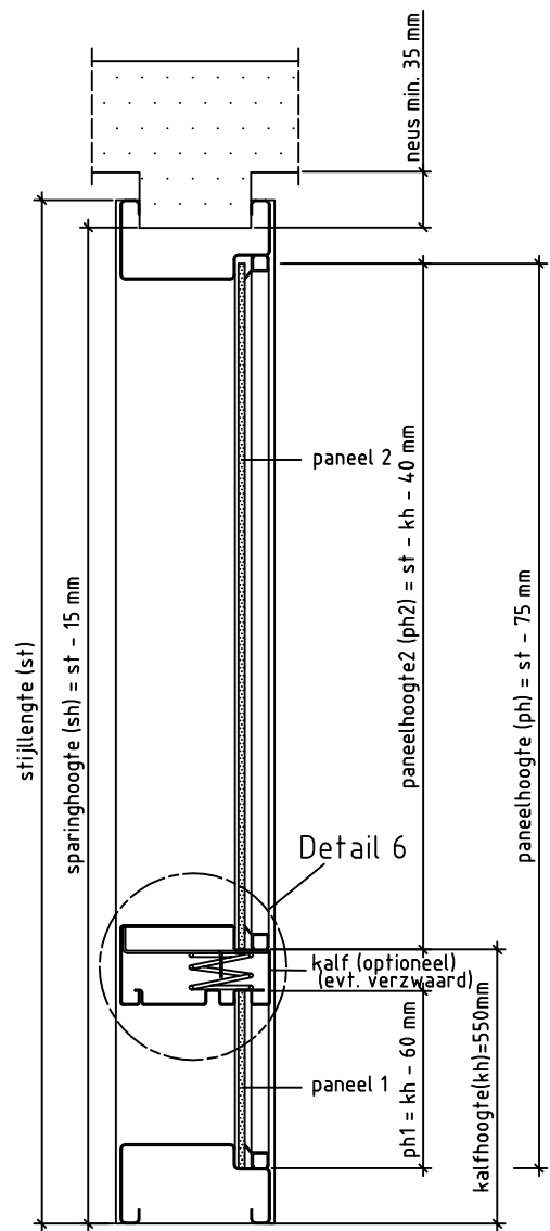
Doorsnede CC
