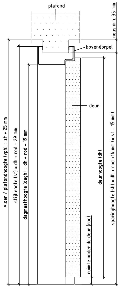
Doorsnede BB
