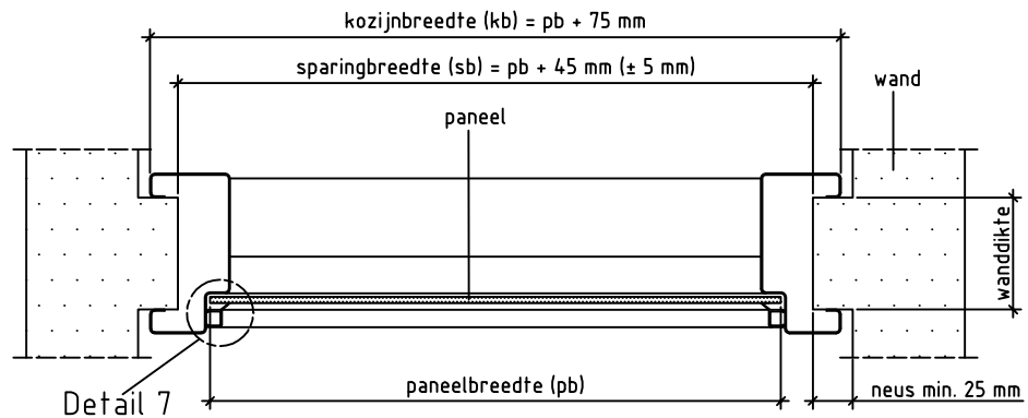
Doorsnede AA
