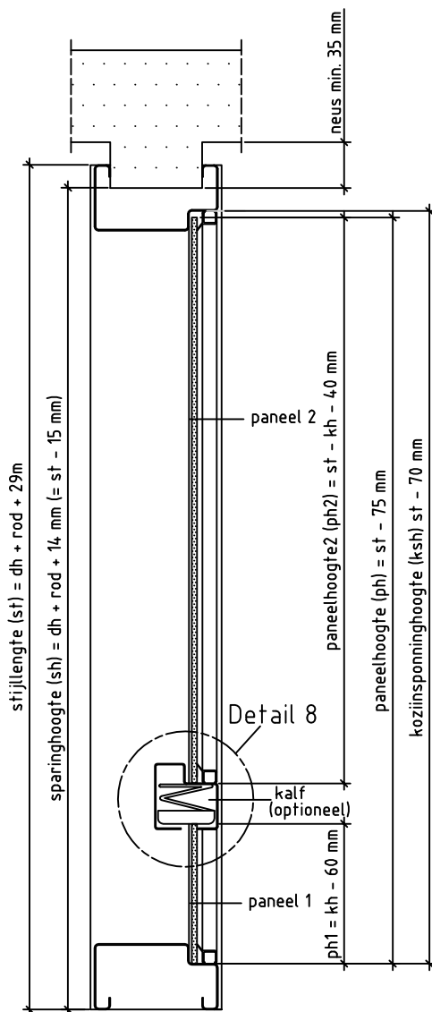
Doorsnede BB
