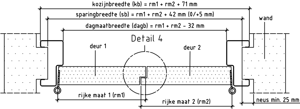
Doorsnede AA
