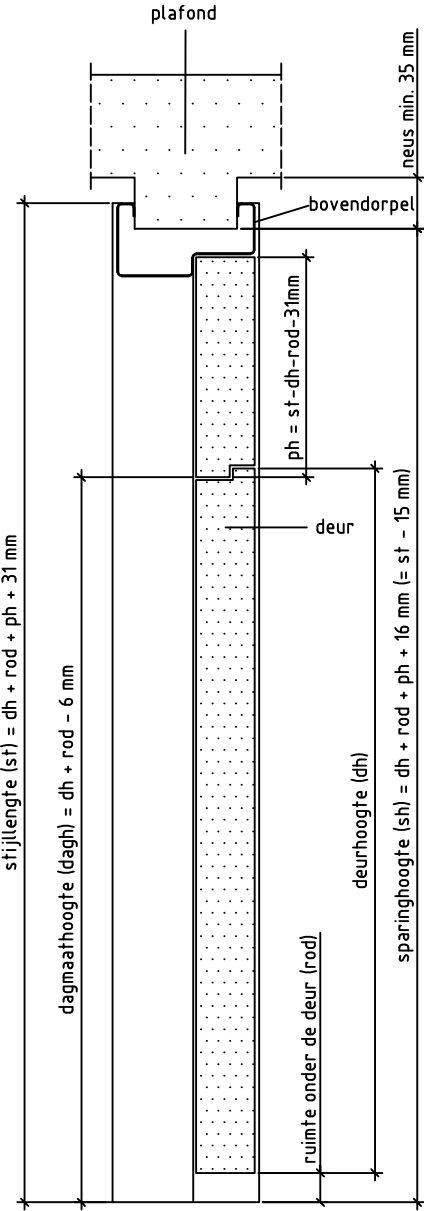
Doorsnede BB
