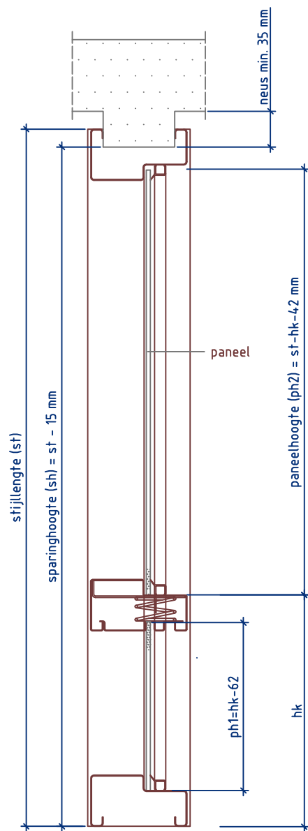
Doorsnede CC
