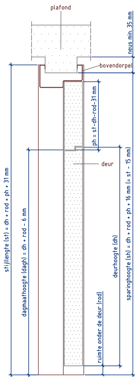
Doorsnede BB
