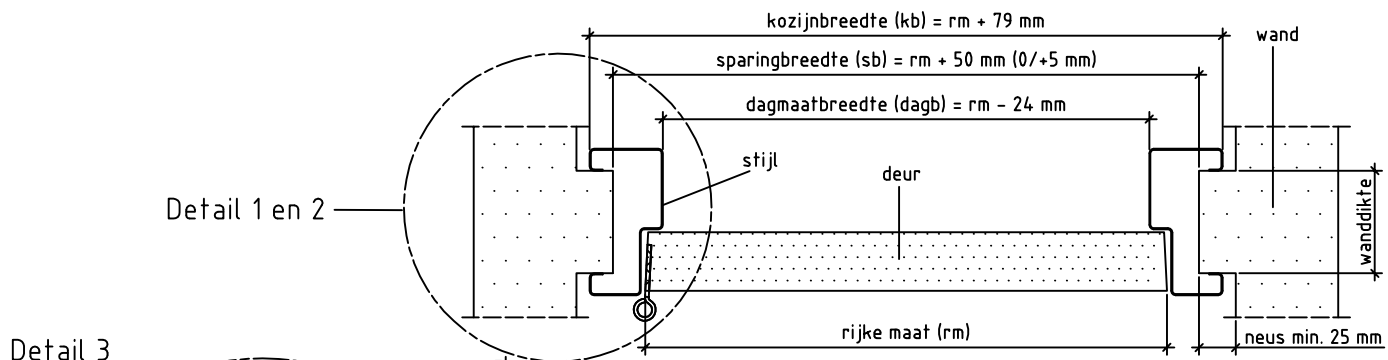
Doorsnede AA
