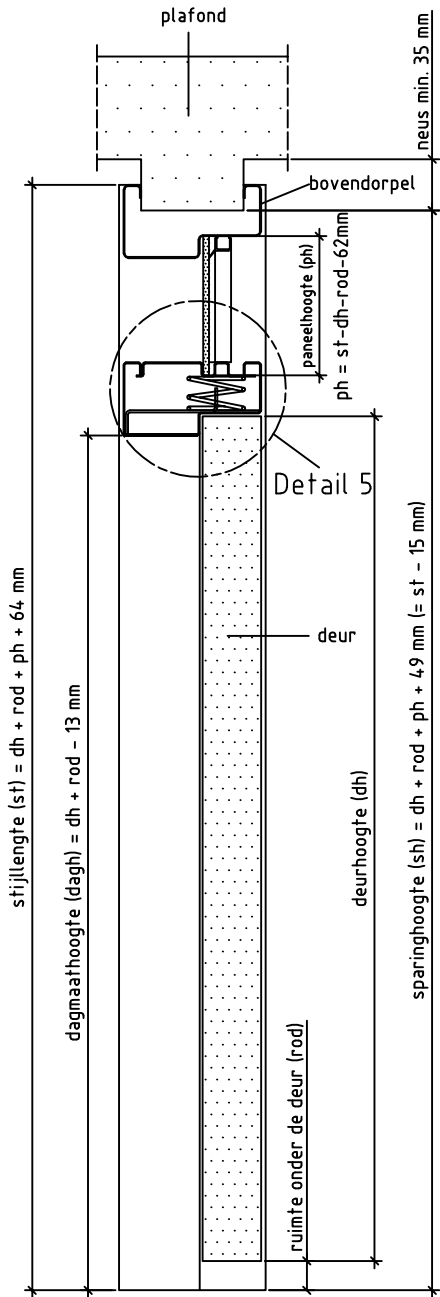
Doorsnede BB
