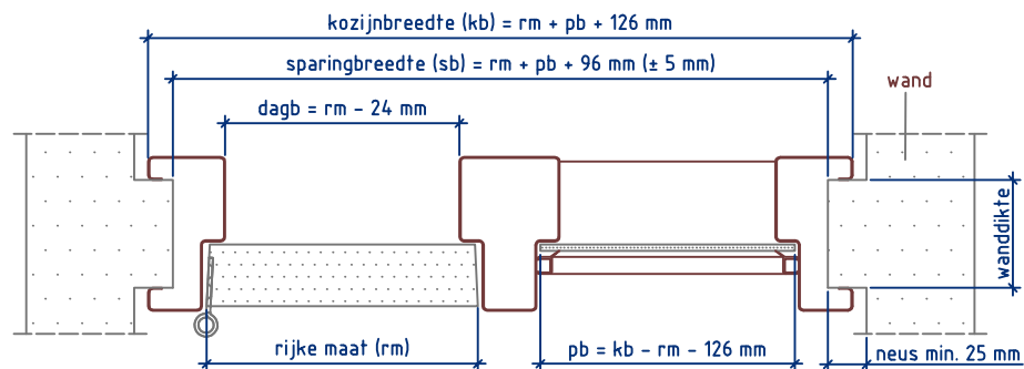
Doorsnede AA
