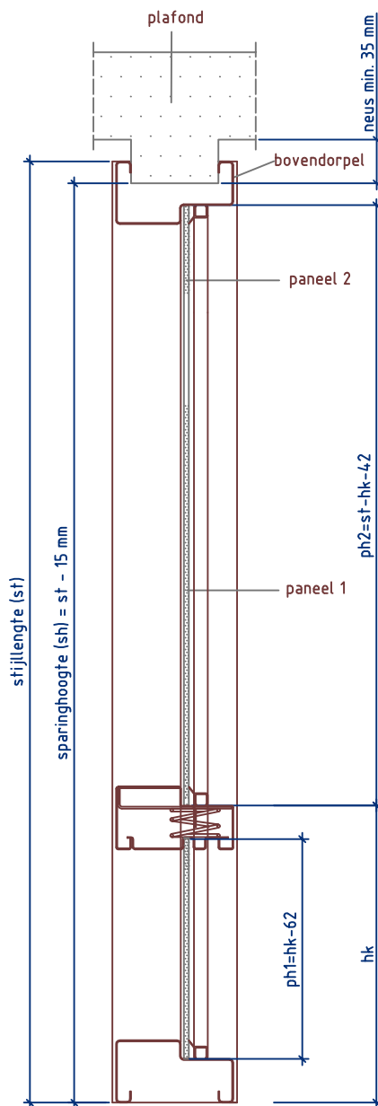
Doorsnede CC
