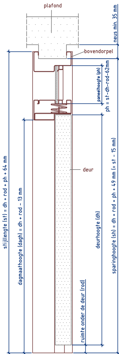
Doorsnede BB
