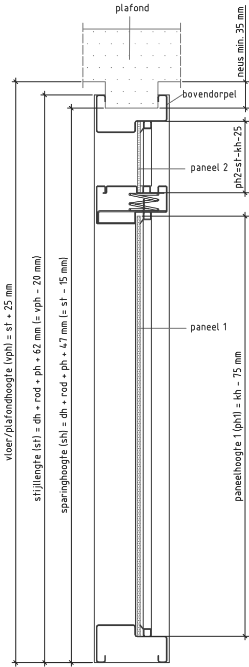
Doorsnede BB
