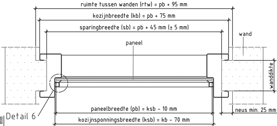
Doorsnede AA
