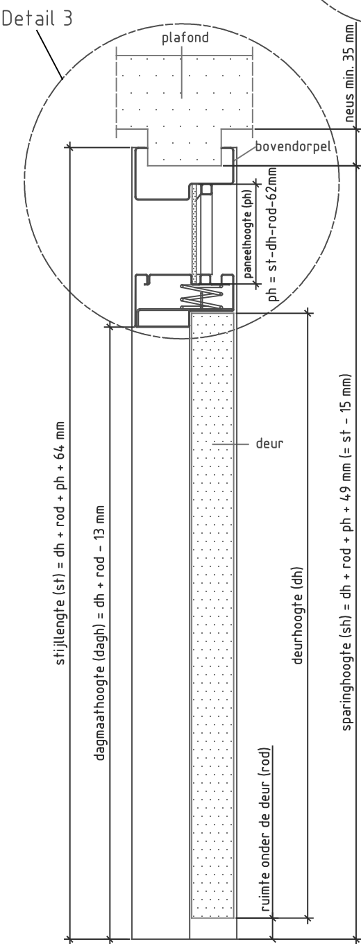
Doorsnede BB
