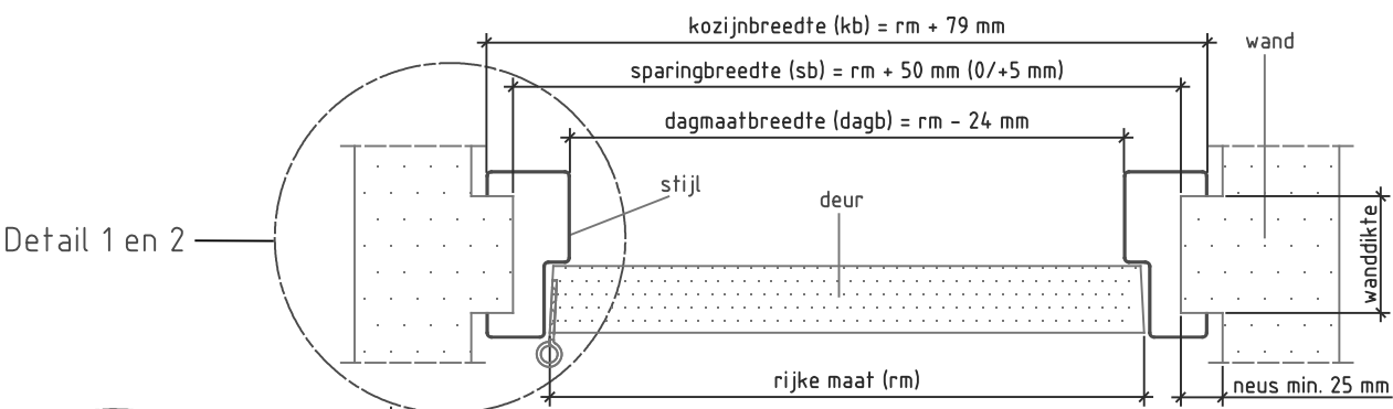
Doorsnede AA
