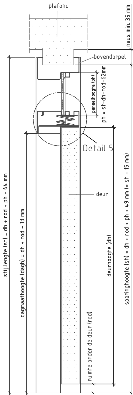
Doorsnede BB
