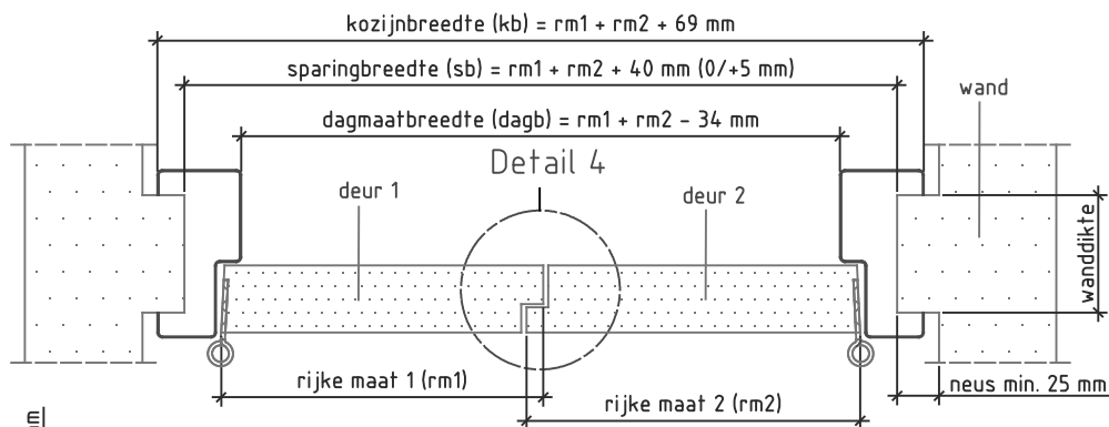
Doorsnede AA
