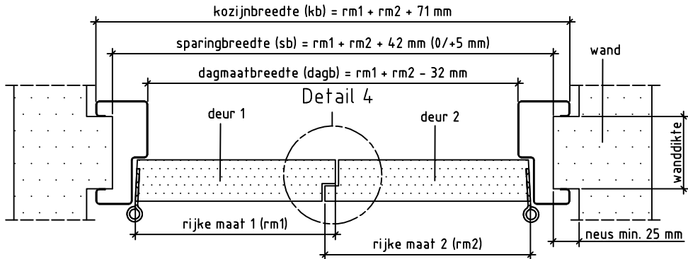
Doorsnede AA
