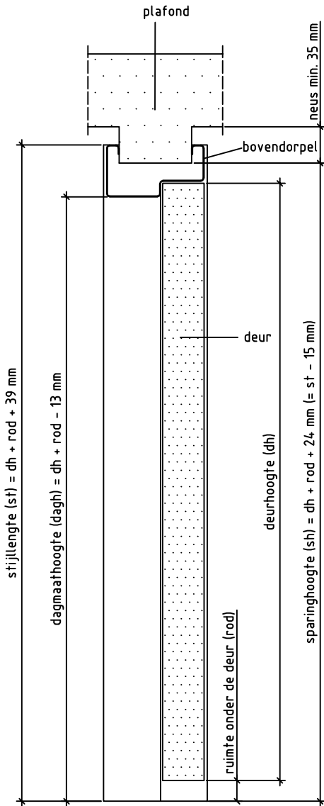
Doorsnede BB
