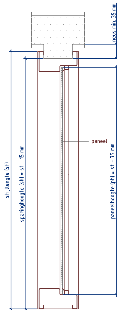
Doorsnede CC
