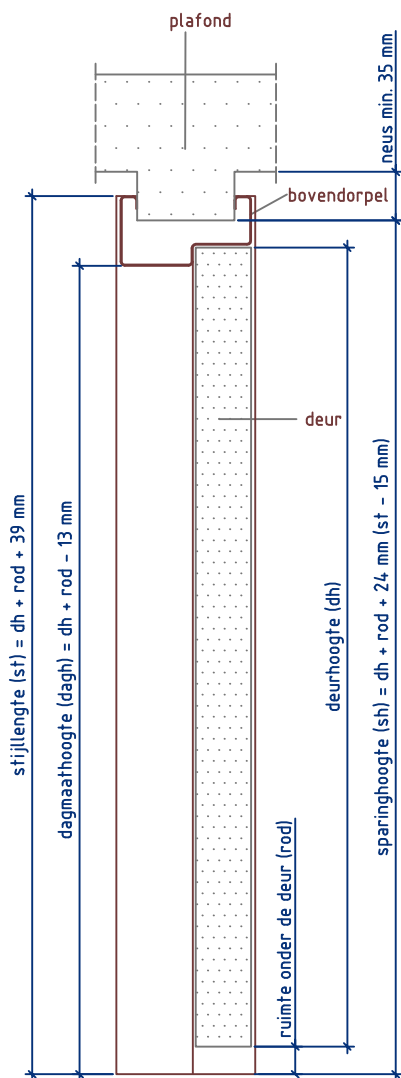
Doorsnede BB
