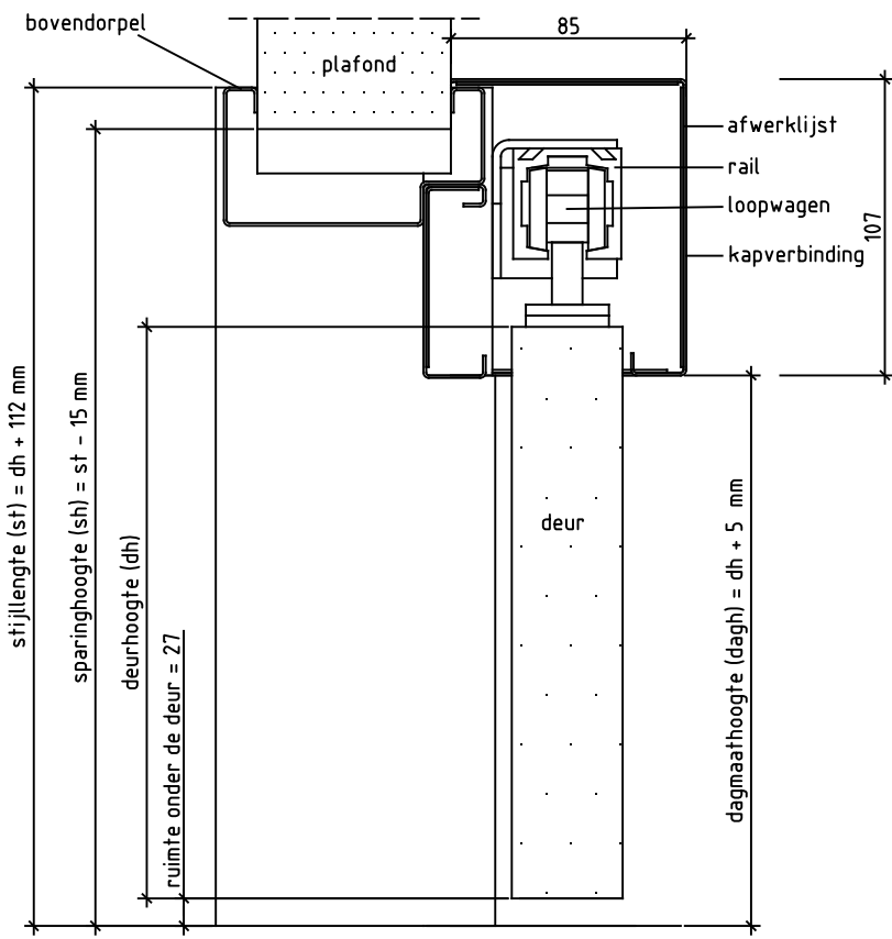
Doorsnede CC
