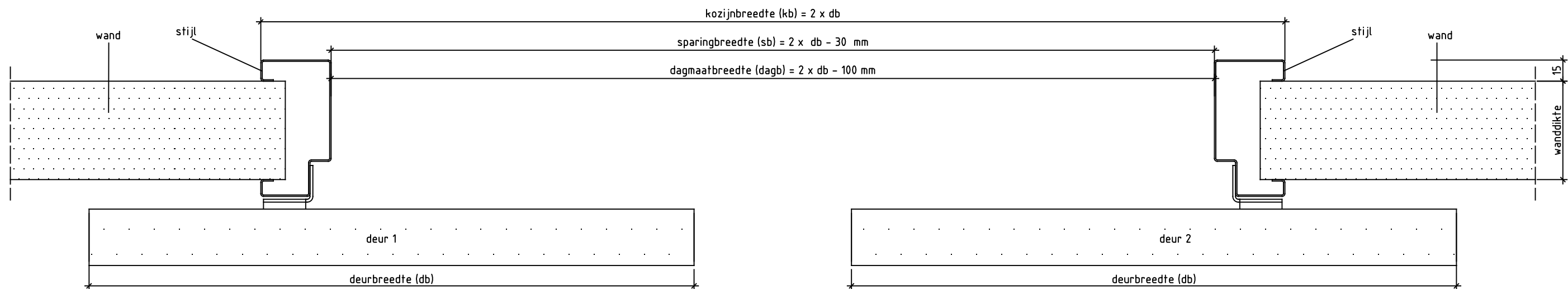
Doorsnede AA
