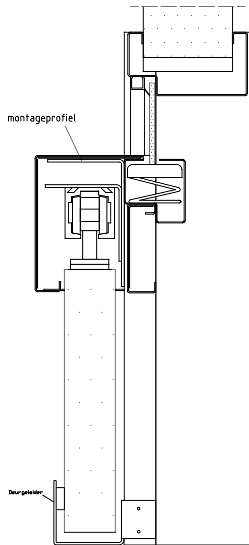
Doorsnede BB
