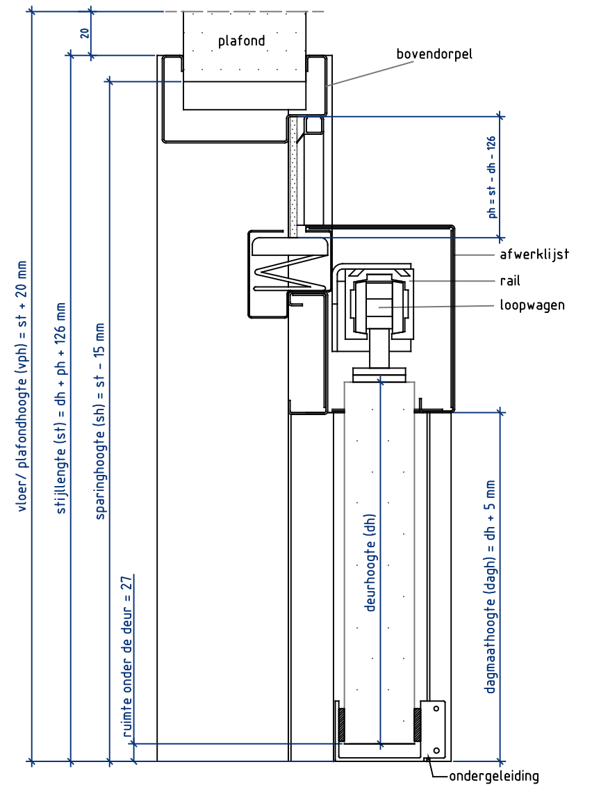
Doorsnede CC
