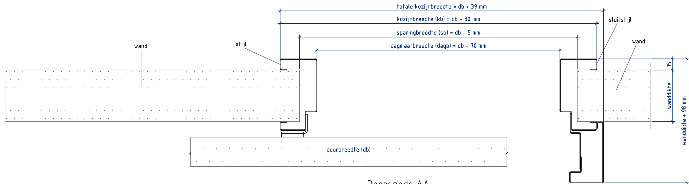
Doorsnede AA
