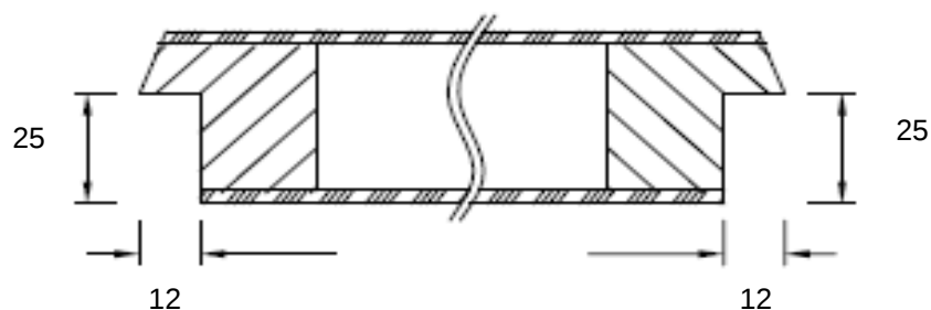
Opdek Schuin (standaard)
