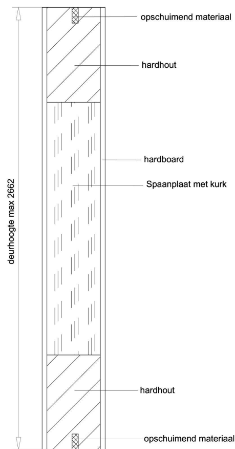
Doorsnede BB
