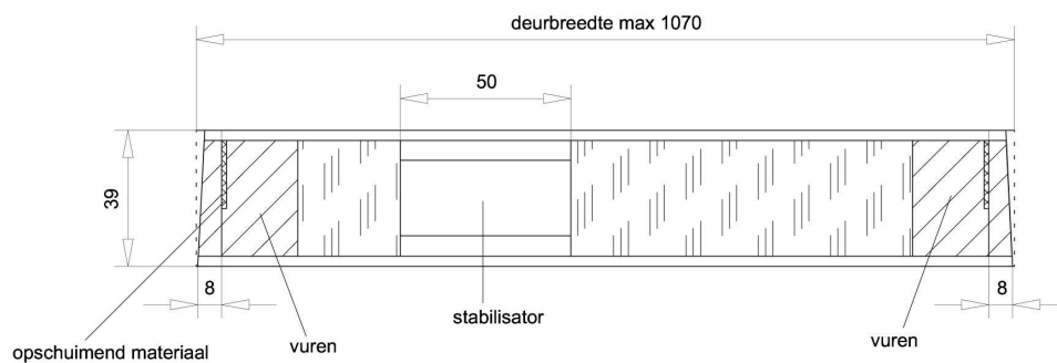
Doorsnede AA
