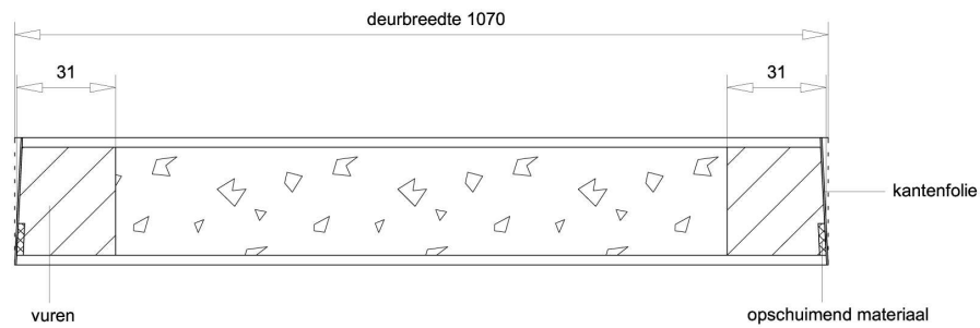
Doorsnede AA
