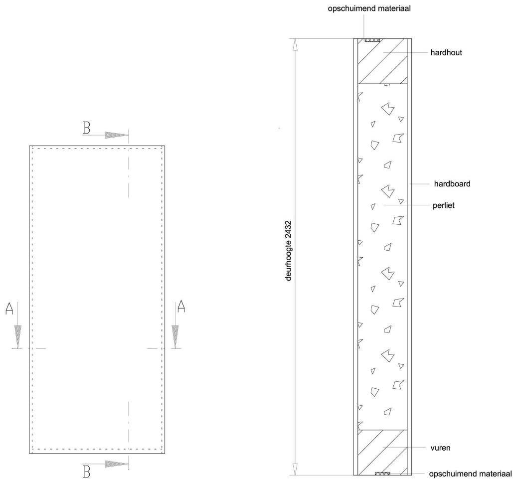
Doorsnede BB
