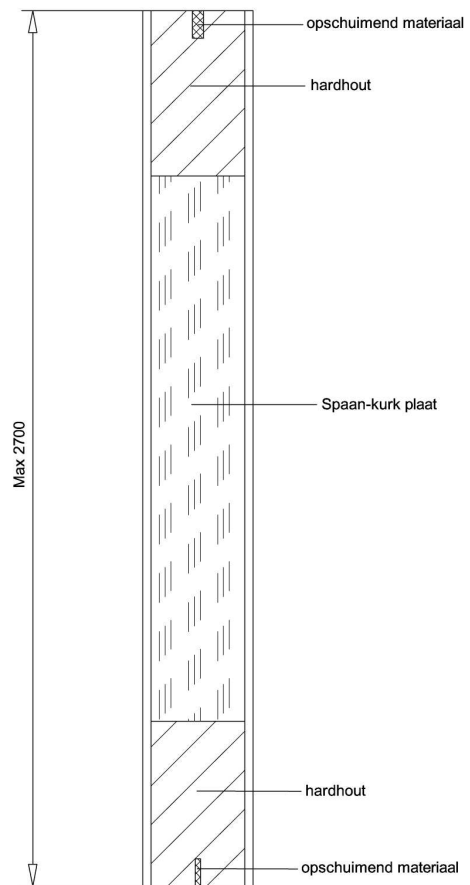
Doorsnede BB
