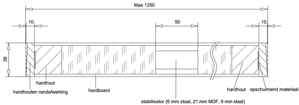
Doorsnede AA
