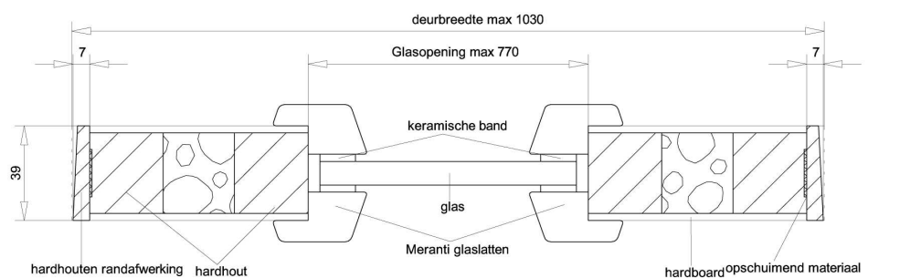
Doorsnede AA
