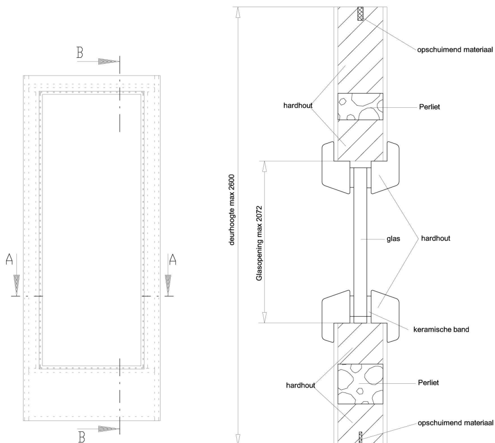
Doorsnede BB
